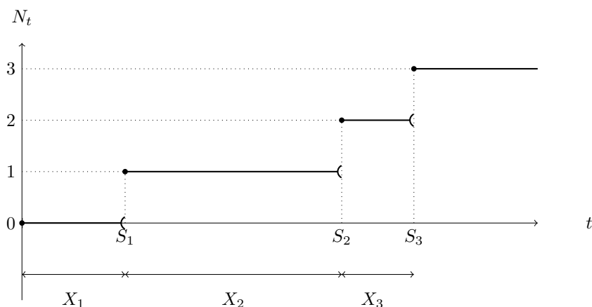
FIGURE 1 – Exemple de réalisation de N_t en fonction de t .
